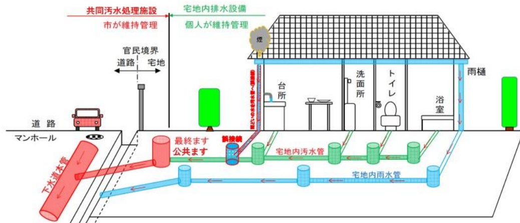
分流方式一般図(誤接続)
